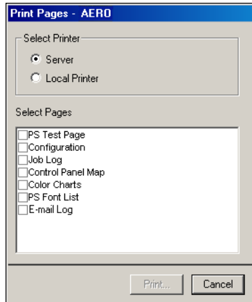
Server options
