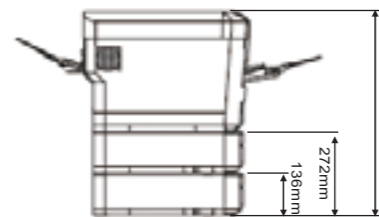
(标配纸盒 + 选配纸盒产品尺寸图)
