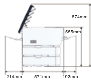
(标配纸盒 + 选配纸盒产品尺寸图)
